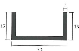
U 2.0×30×15 ○ シルバー (B2) ○ シルバークリア (有) ● ブラック (消)
