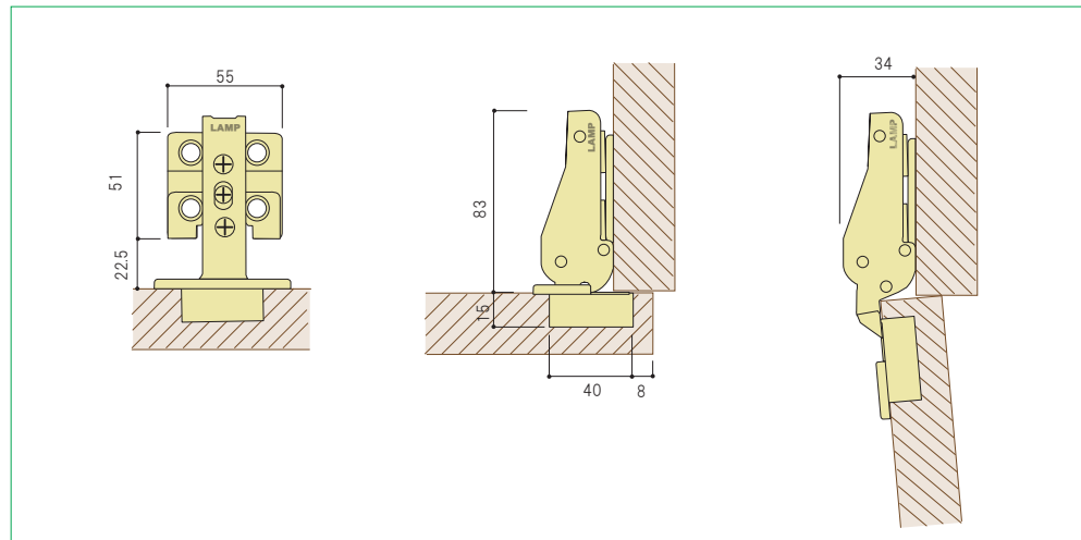
J95-P6T マウンティングプレート付き
