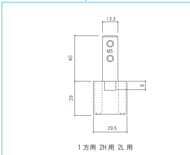
コネクター
