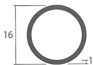
1.0×16 ○ シルバー B2
