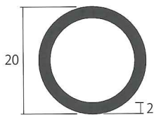
2.0×20 ○ シルバー B2
