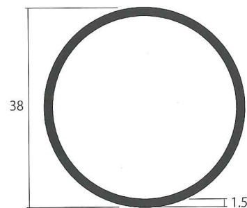
1.5×38 ○ シルバー B2
